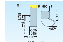
單位：毫米 黃色空間指的是散熱空間 Unit: mm Yellow spaces mean heat space
