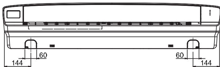
&lt;Rear View&gt;
