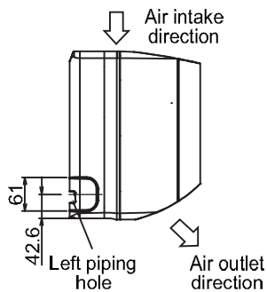
&lt;Side View&gt;
