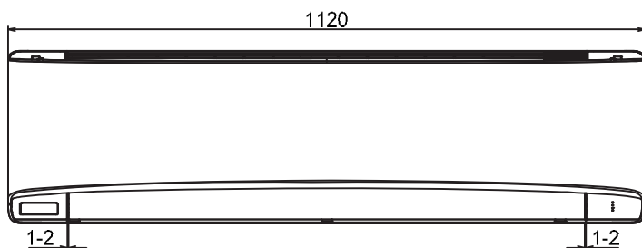
&lt;Front View&gt;
